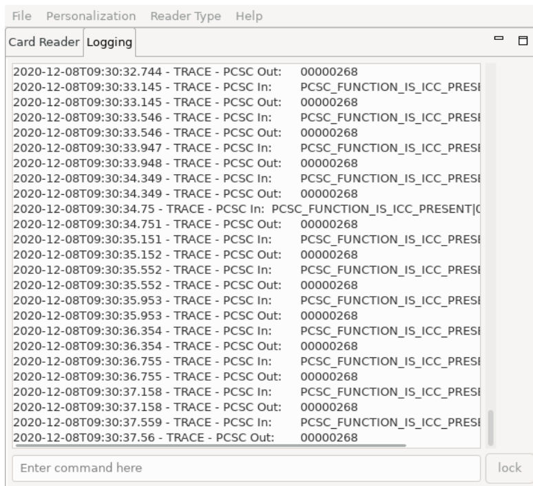
Abbildung 4: PersoSim Konsole
