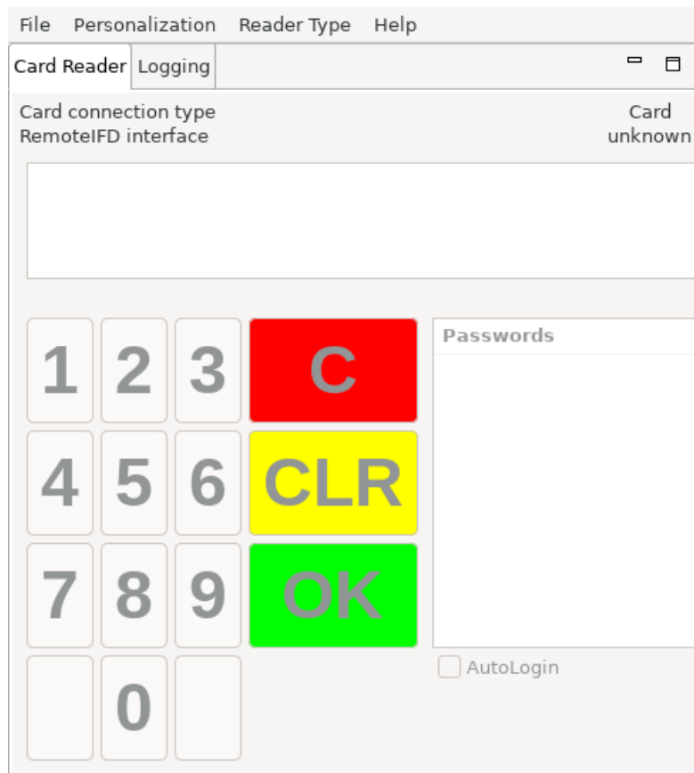
Abbildung 1: PersoSim Hauptfenster
